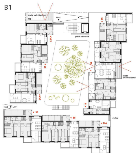
TLORIS 1. NADSTROPJA_OBJEKT B1 m_1:200
