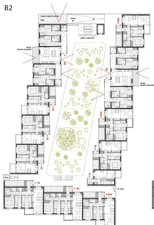
TLORIS 1. NADSTROPJA_OBJEKT B2 m_1:200
