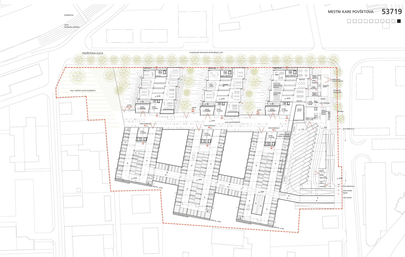
SITUACIJA - NIVO SOSESE - SPODNJE ULICE - 1. KLETI m. 1:500
