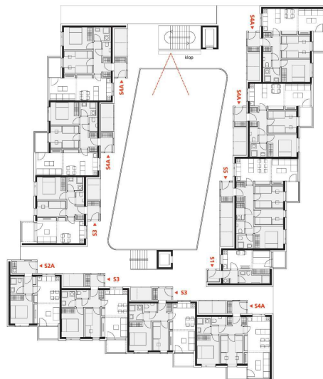
TLORIS 2.-6. NADSTROPJA_OBJEKT A3 m_1:200
