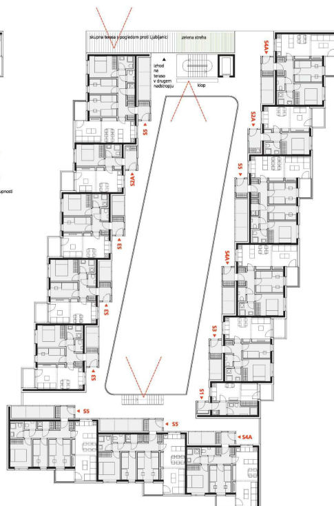
TLORIS 2. NADSTROPJA_OBJEKT B2 m_1:200
