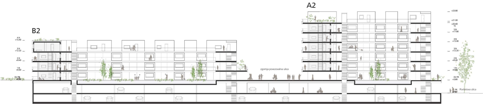
PREREZ C-C m_1200
