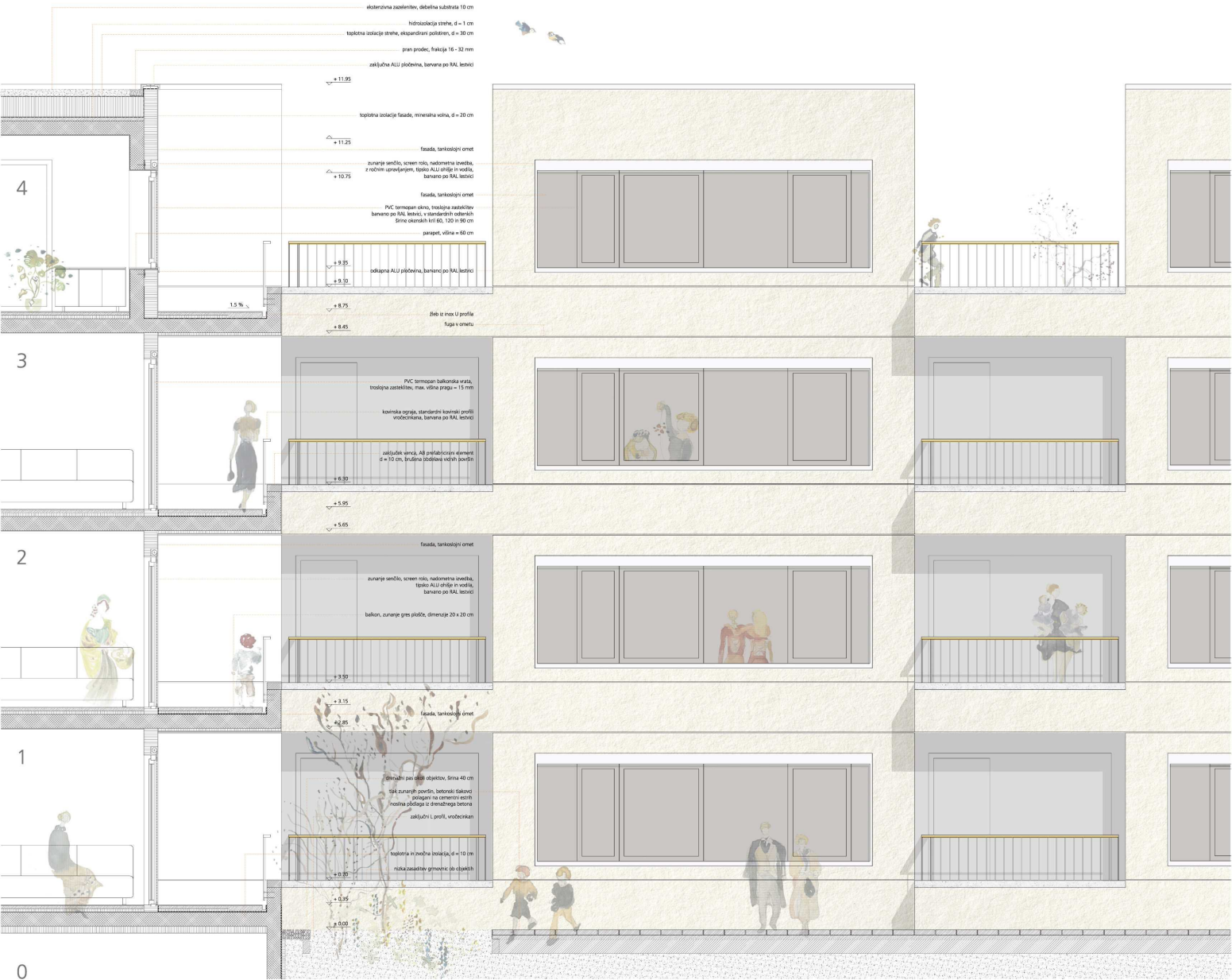
FASADNI PAS_ZUNANJE DVORIŠČE m_125
