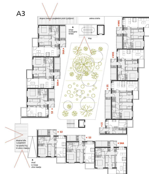
TLORIS 1. NADSTROPJA_OBJEKT A3 m_1:200
