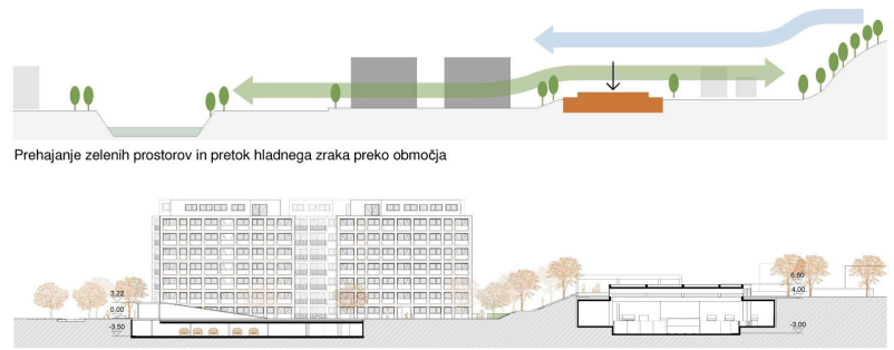
Prečni prerez | 1 : 500
