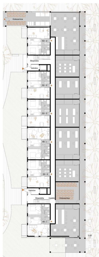
Blok B2 - tloris pritličja | 1 : 200
