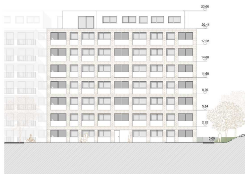
Blok A - urbana fasada | 1 : 200
