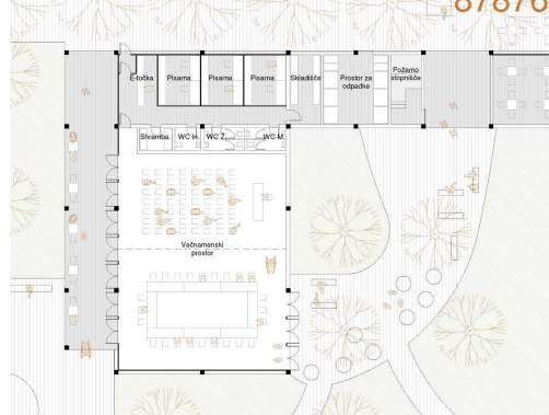
Tloris pritičja - javni program | 1 : 200
