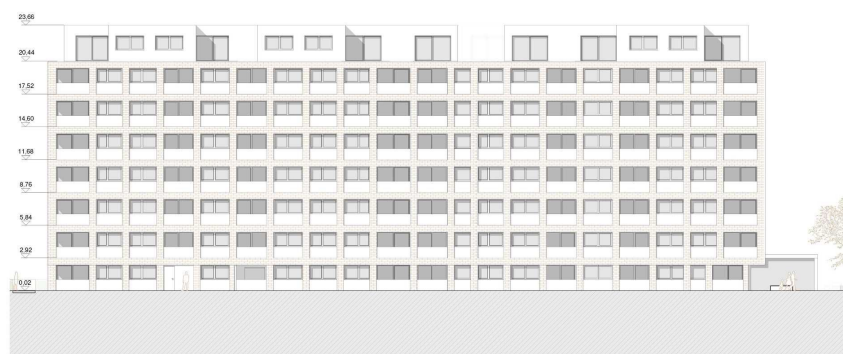
Blok B - urbana fasada | 1 : 200
