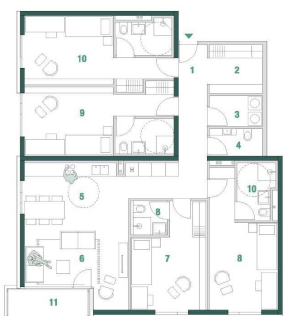
KATALOG STANOVANJA - BIVALNA ENOTA, M 1:100
