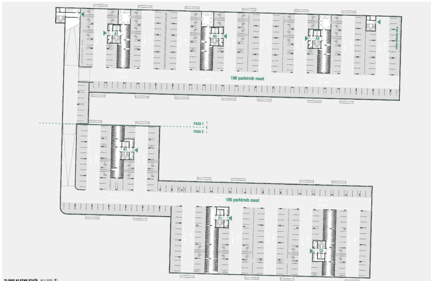
TLORIS KLETNE ETAŽE, M 1:500
